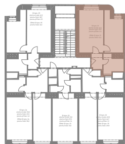
půdorys podlaží
